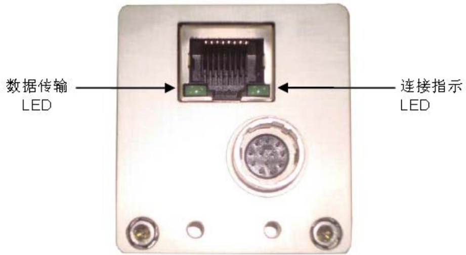
相机网口指示灯
